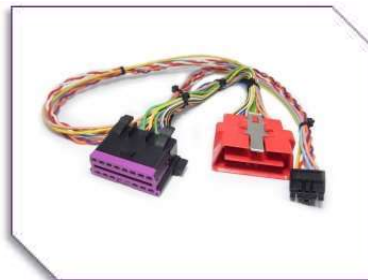
OBD-II Cable
