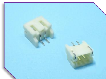
E17 2.00mm JST PH Series
