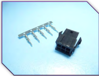
E32-H1 3.00mm Micro Fit Molex 43025
