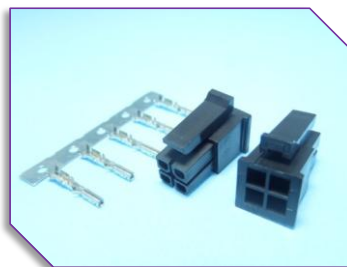
E32-H2 3.00mm Micro Fit Molex 43025
